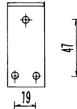
取付金具3-φ6
